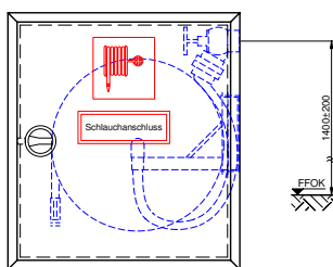
Anschluss auf rechter Seite
