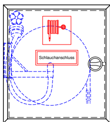
Anschluss durch Rückwand links
