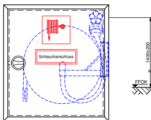
Anschluss durch Rückwand rechts
