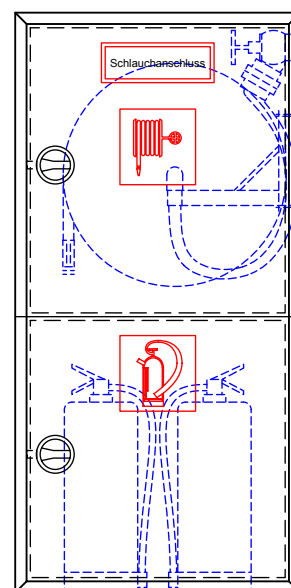
Ausführung DK - kombinierter Wandschrank mit Schlauchhaspel/Armatur und Raum zum Einstellen von zwei Feuerlöschern
